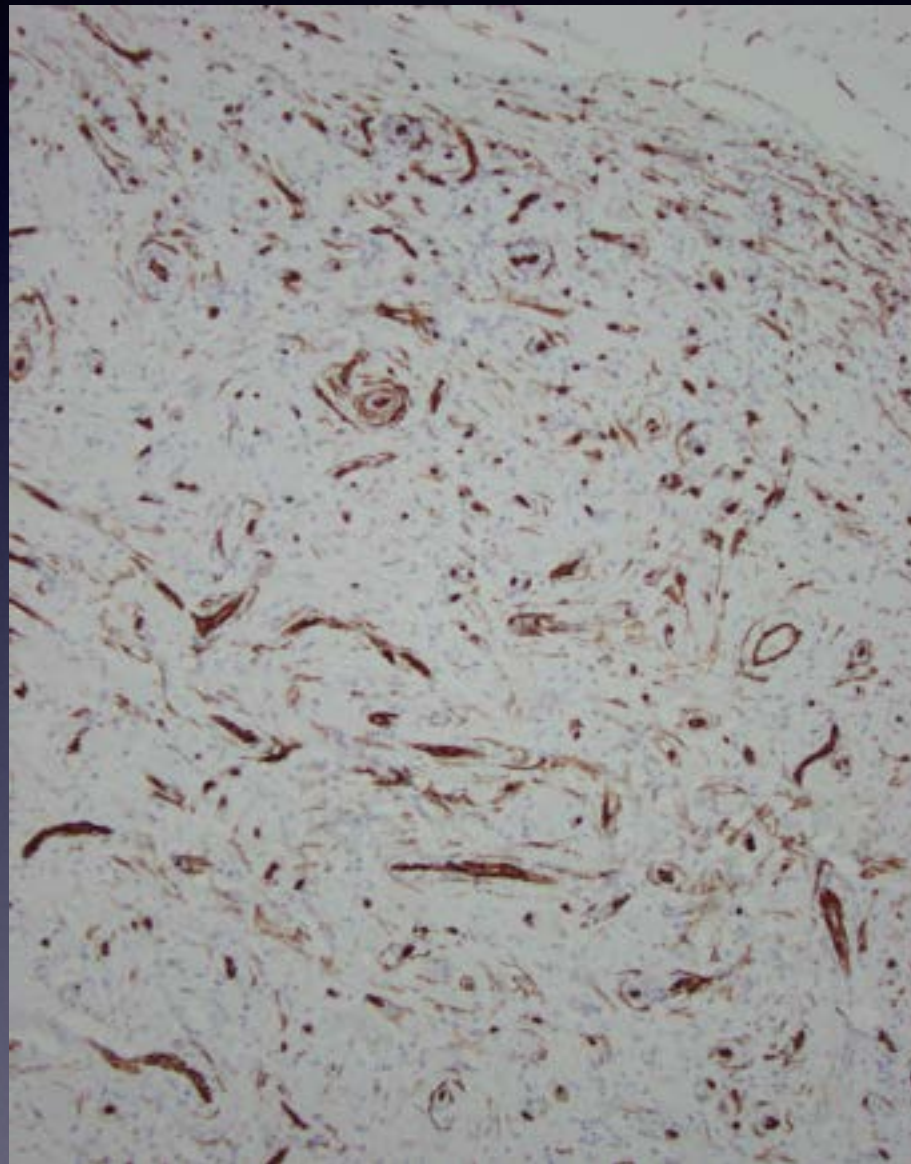
CD34
