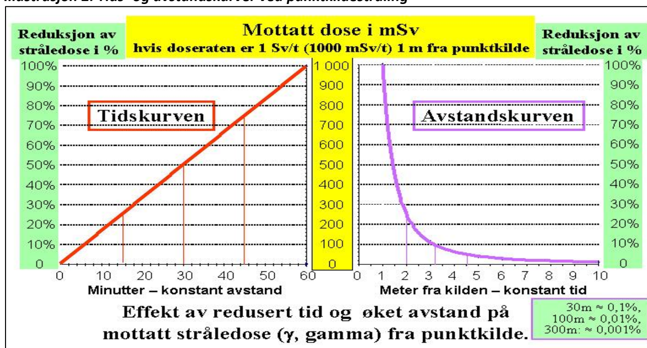
Illustrasjon 2: Tids- og avstandskurver ved punktkildestråling
